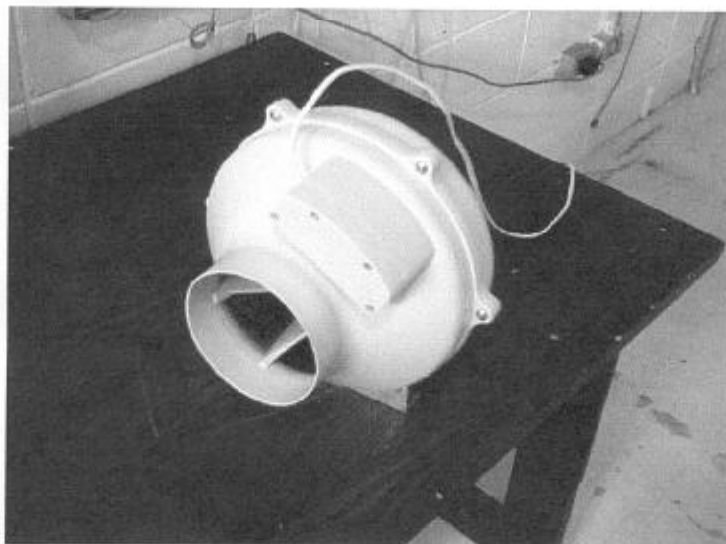
Figura 1 – Ventilador ensaiado
